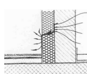
obróbki blacharskie poprowadzone pod tynk izolację termiczną
