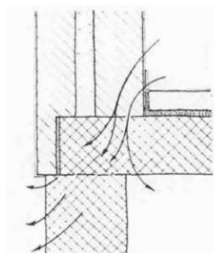
przeście izolacji wewnętrznej na zewnętrzna lub pośrednią
