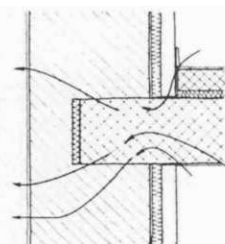
izolacja wewnętrzna przy zakotwieniu stropu w ścianie
