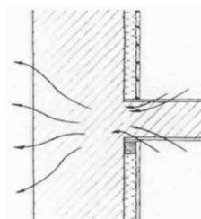
monolityczne połączenie płyty stropowej ze ścianą
