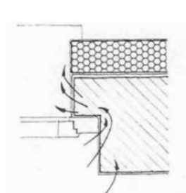
nie ocieplone ościeża i nadproża
