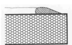
uformować zaprawę w kształcie pryzmy, przeciągając szpachelką pod kątem 45°
