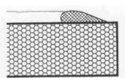
uformować zaprawę w kształcie przyny, przeciągając szpachelką pod kątem 45°
